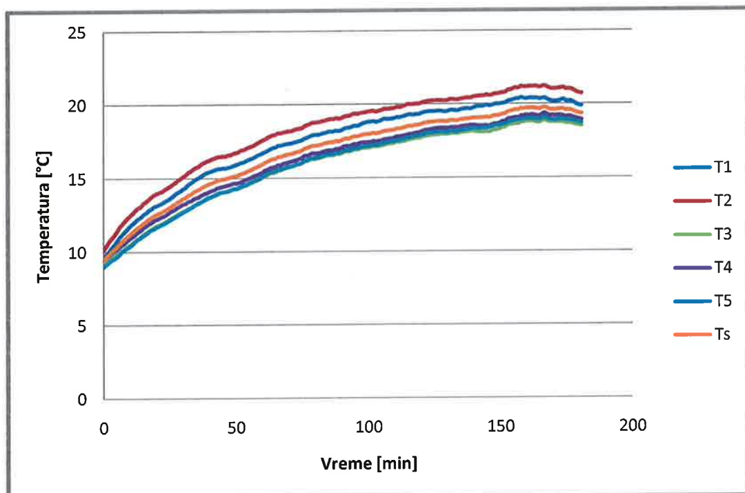
Slika 1 - Vremenske promene temperatura na neizloženoj površini uzorka
