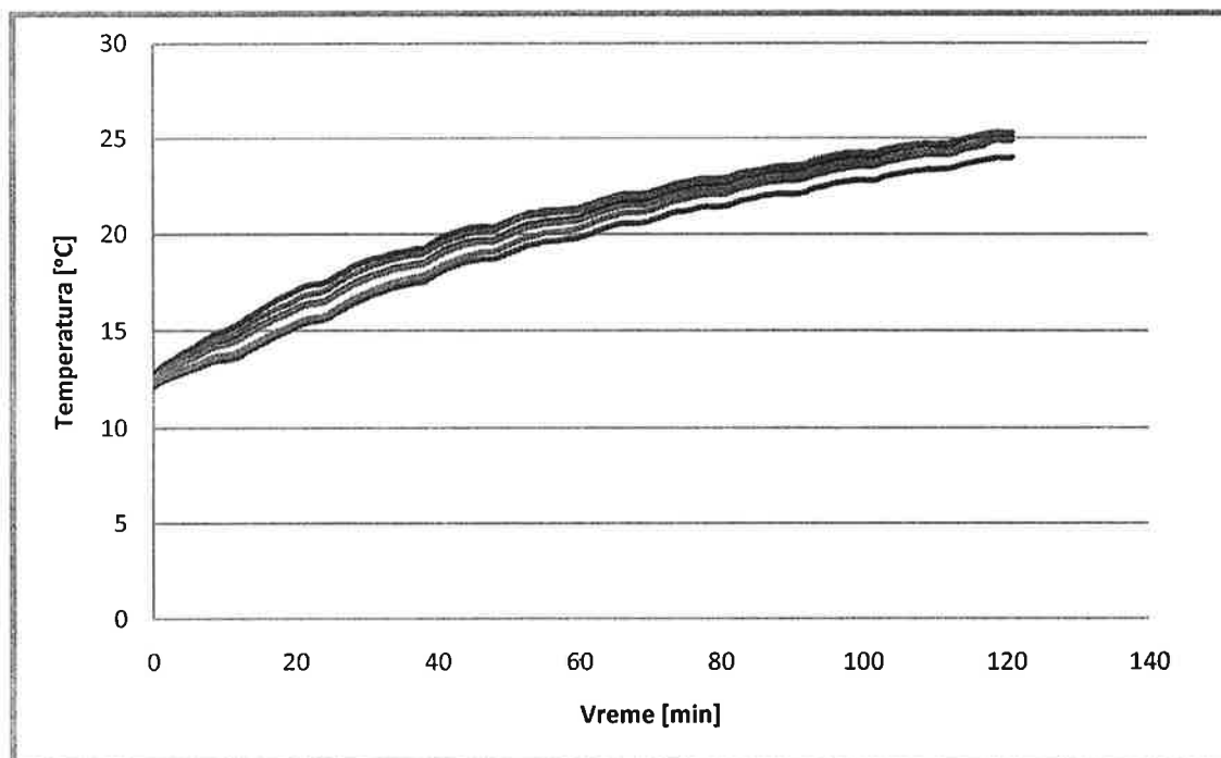
Slika 1 - Vremenske promene temperatura na neizloženoj površini uzorka
